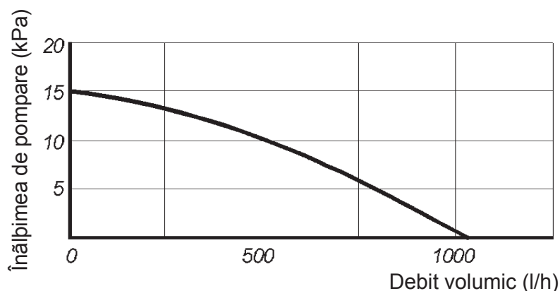
Caracteristica hidraulică rezultantă a ansamblului pompă – schimbător electric EH 3
